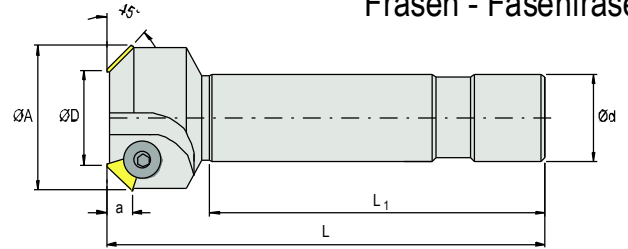
Parmak Freze Milling - Chamfer Mill Fräsen - Fasenfräsen
